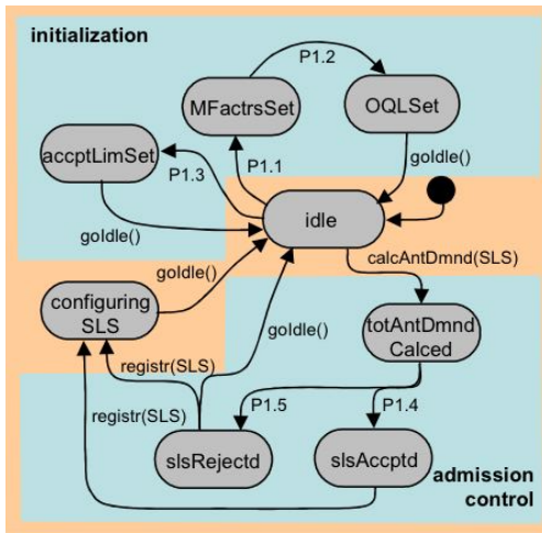
Fig. 2. SLS-S module behavior.
