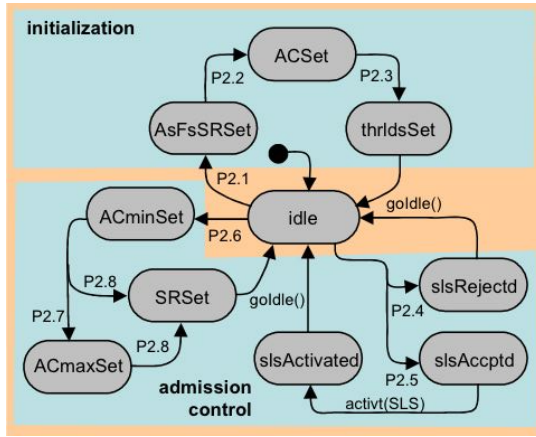
Fig. 3. SLS-I module behavior.
